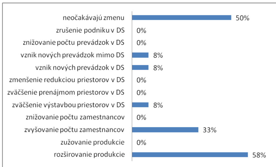
Obr. č. 7: Očakávaný vývoj podniku v najbližších troch rokoch
