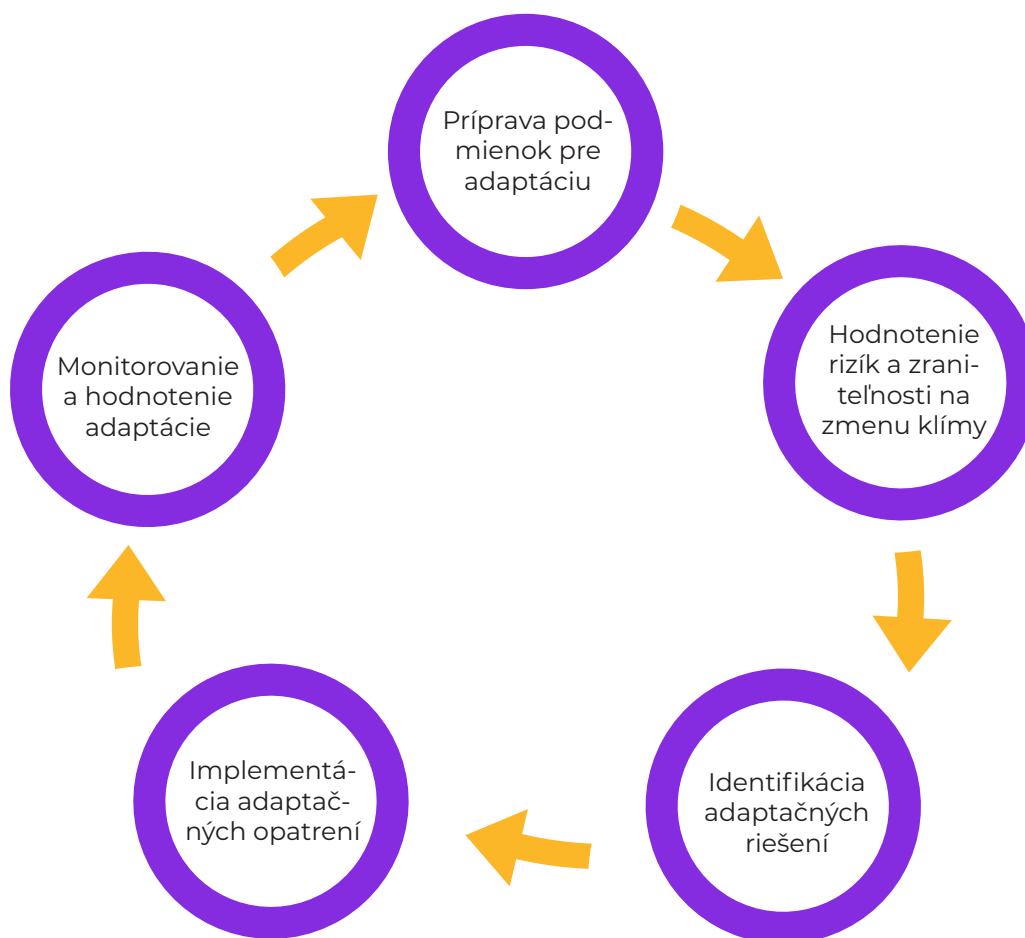
Obr. 3: Model proaktívnej adaptácie mesta na zmenu klímy
