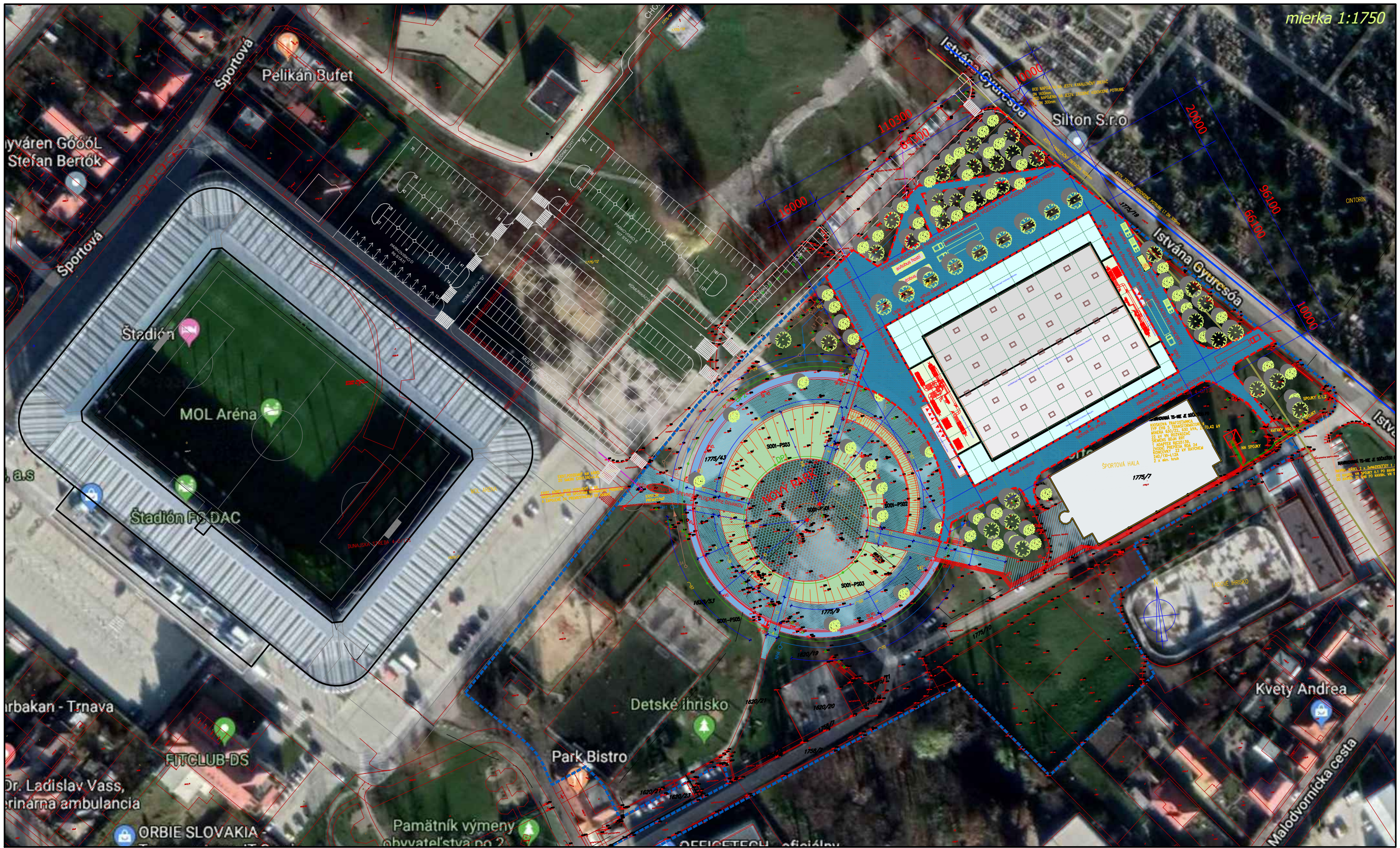
ŠIRŠIE VZŤAHY OSADENIA NOVEJ MULTIFUNKČNEJ ŠPORTOVEJ HALY S PREPOJENÍM NA NOVÉ NÁMESTIE A NA OSTATNÉ KOMUNIKÁCIE MESTA
